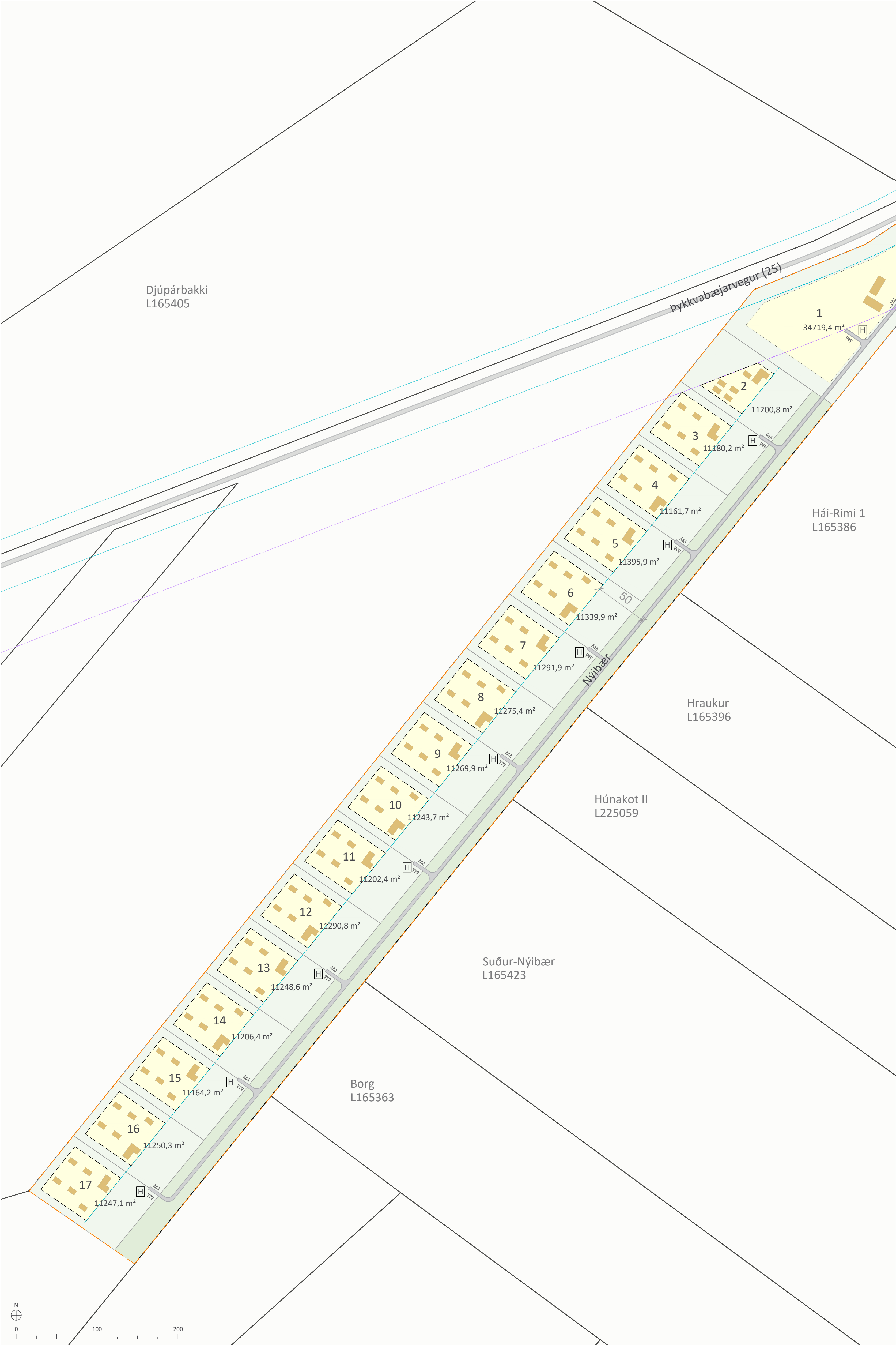
DEILISKIPULAGSUPPDRAÐTÚR 1:2500
