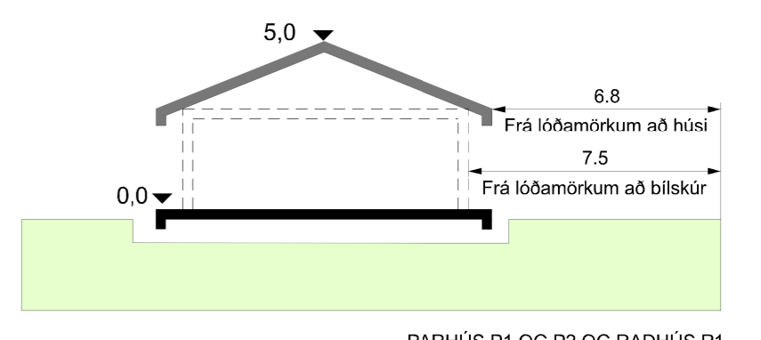
PARHÚS P1 OG P2 OG RADHÚS R1 SKÝRINGARMYND Mkv. 1:200
