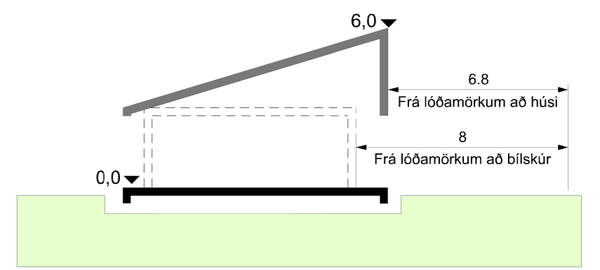
EINBYLIÐSHÚS E1 SKÝRINGARMYND Mkv. 1:200
