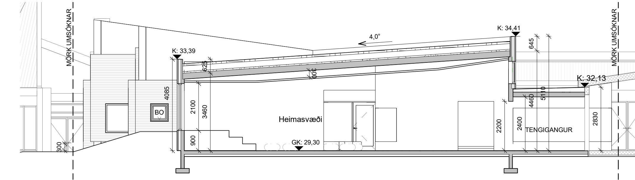
3 ÞVERSNIÐ D-D 1 : 100
