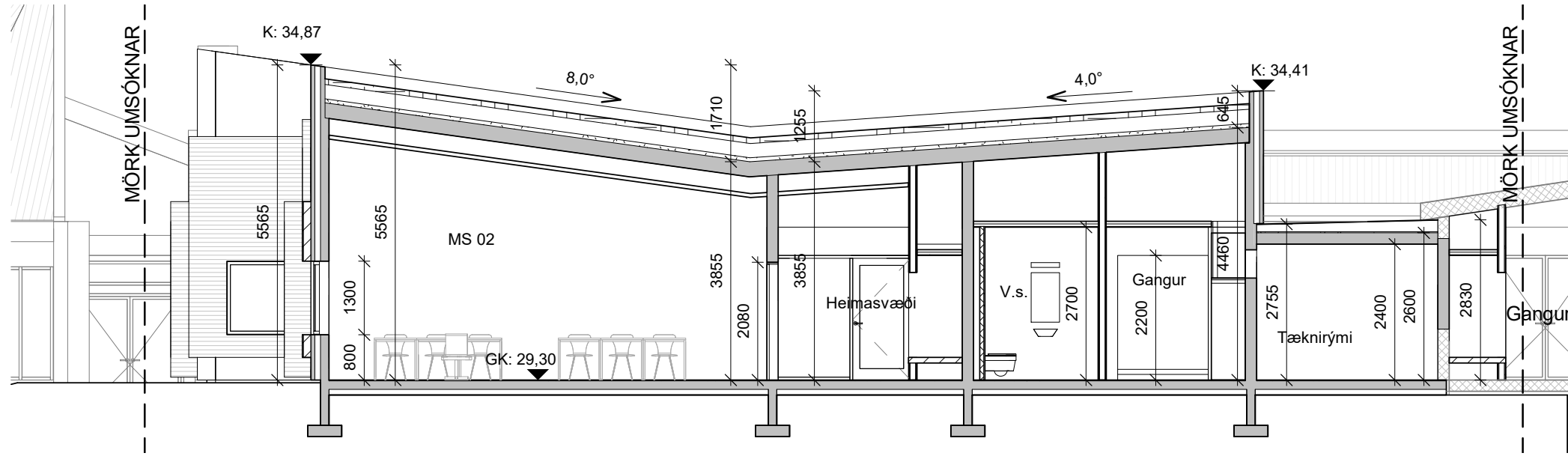
1 ÞVERSNIÐ E-E 1 : 100
