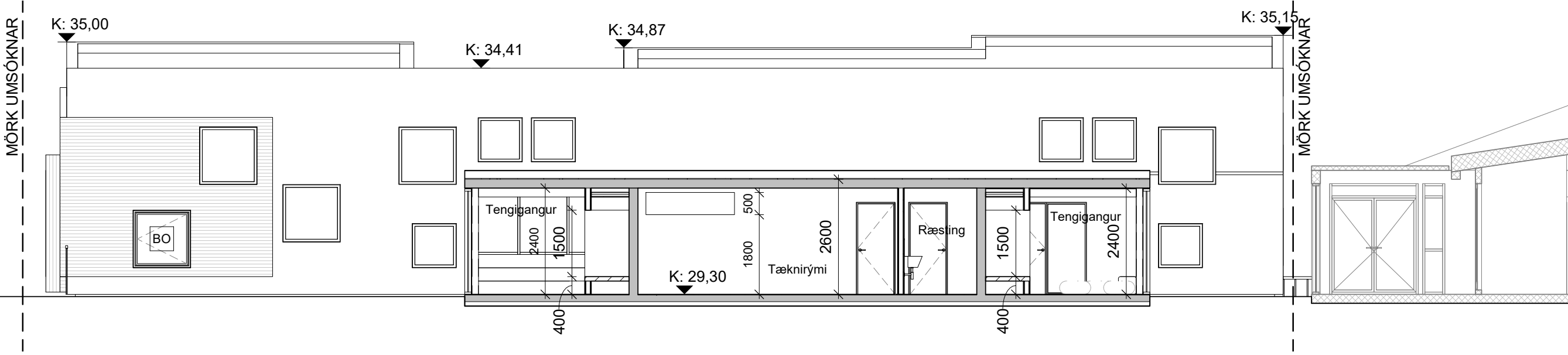
6 LANGSNIÐ B-B (ÁSÝND) 1 : 100
