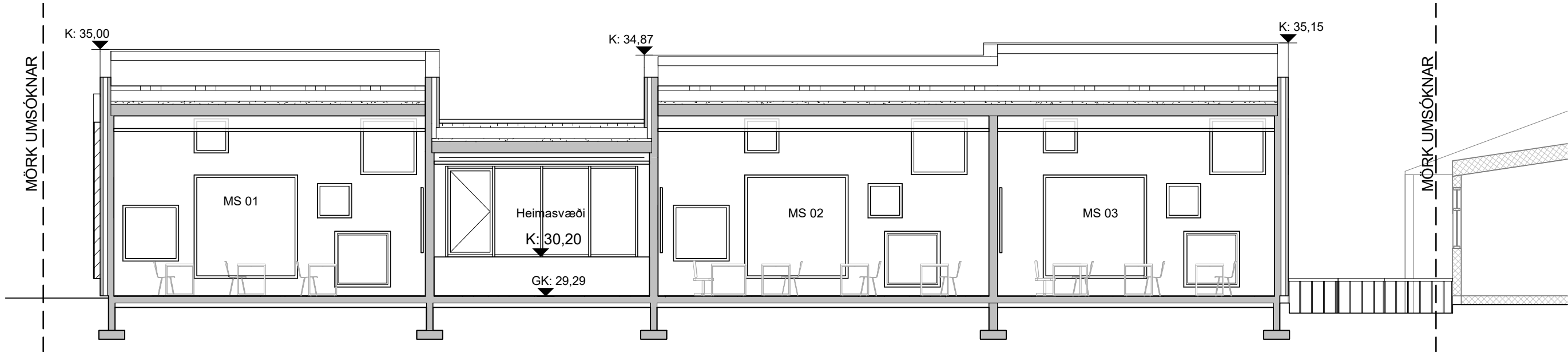
5 LANGSNIÐ A-A 1 : 100
