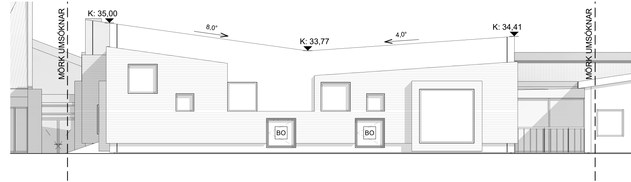
7 ÁSÝND VESTUR 1 : 100
