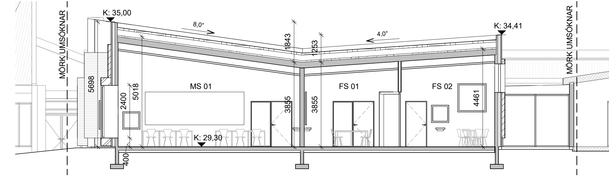
2 ÞVERSNIÐ C-C 1 : 100
