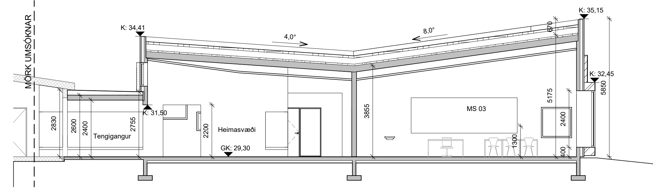
9 ÞVERSNIÐ F-F 1 : 100
