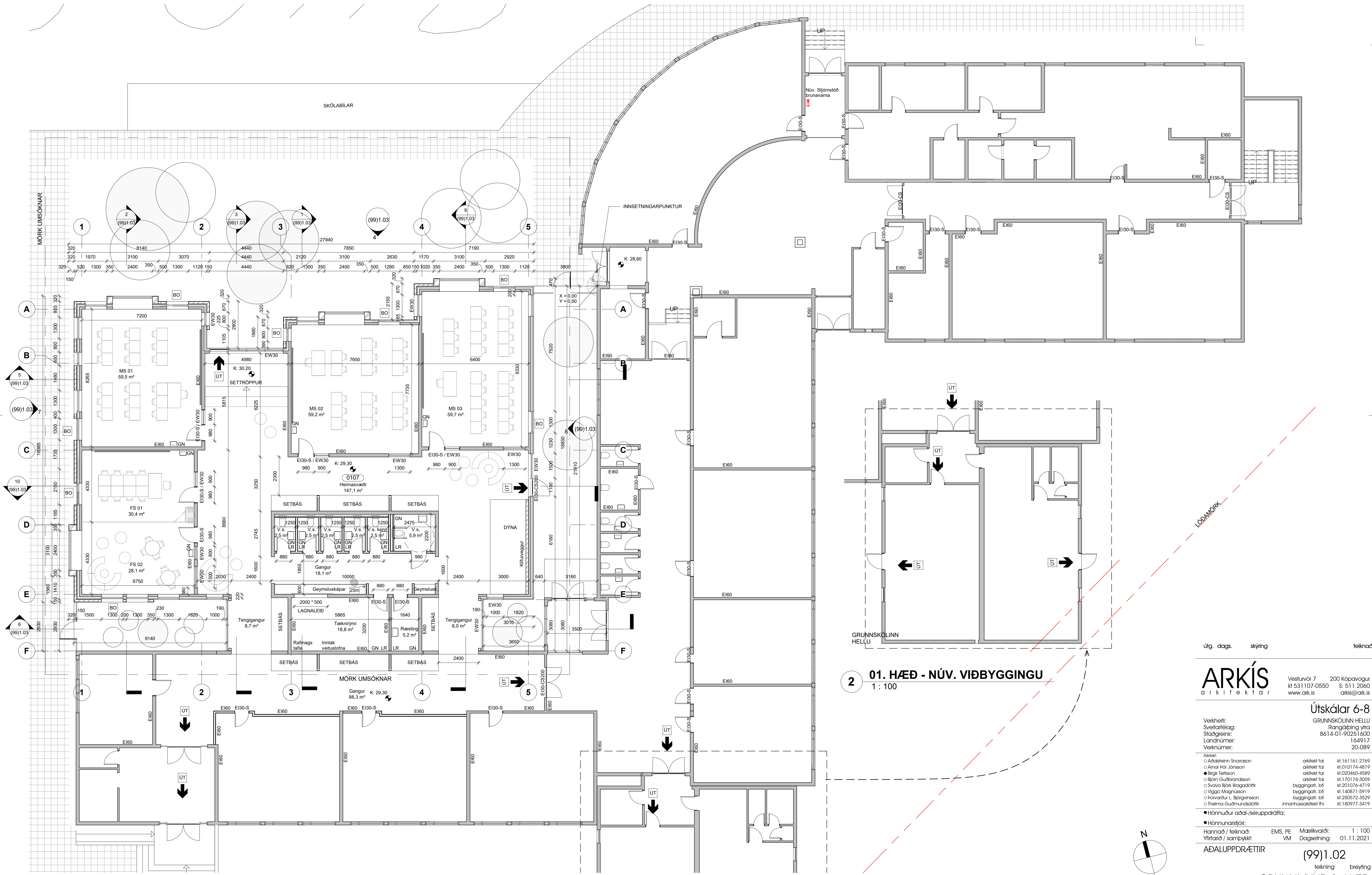
01. HÆÐ 1 : 100
