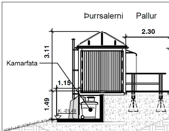
Mynd 5. Dæmi um snið af þurrsalerni.
